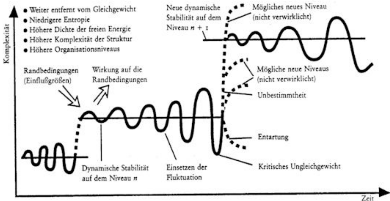
Abb. 2: Bifurkation in einem komplexen System fern vom Gleichgewicht. Fluktuationen, die über die vorgegebenen Randbedingungen hinausgehen, erzeugen eine kritische Instabilität mit nachfolgendem Chaos. Ein nicht determinierter Übergang (eine Bifurkation des Entwicklungsweges des Systems) vollzieht sich, indem sich das dynamische Verhalten des Systems bei Erreichen des kritischen Ungleichgewichts umstrukturiert und auf ein neues Stabilitätsniveau übergeht.
